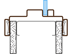
1P Sill Glazing
